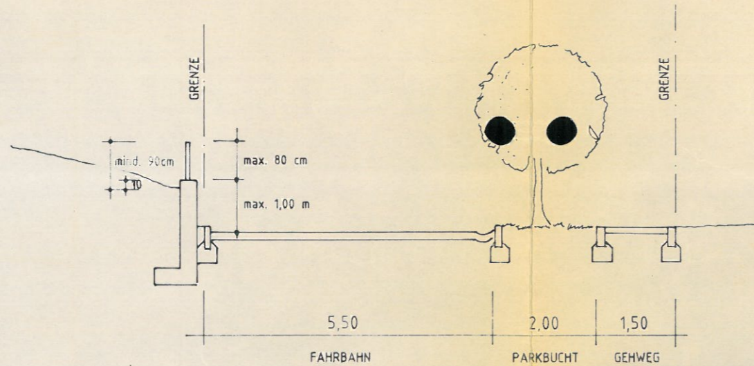
REGELQUERSCHNITT 1 GÜLTIG FÜR STRASSE A
