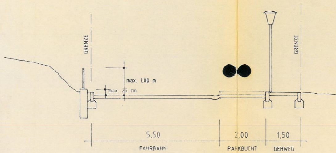
REGELQUERSCHNITT 1 GÜLTIG FÜR STRASSE A
