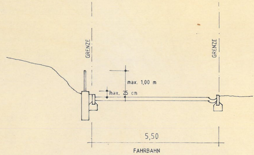
REGELQUERSCHNITT 2 GÜLTIG FÜR STRASSEN B,C,D
