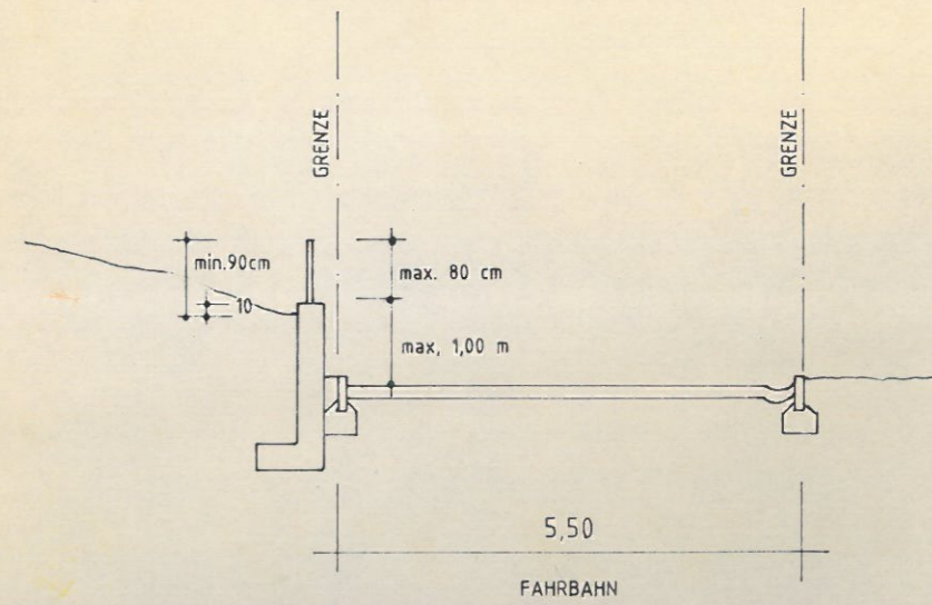
REGELQUERSCHNITT 2 GÜLTIG FÜR STRASSEN B,C,D
